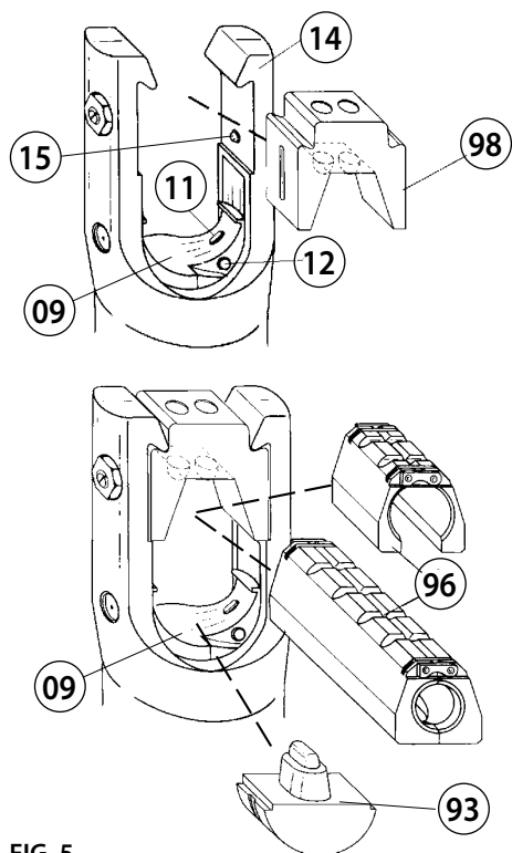
FIG. 5 DIE INSERTION - INSERTION DES MATRICES - EINSETZEN PRESSEINSÄTZE - INSERCIÓN DE LAS MATRICES - INSERIMENTO MATRICI
