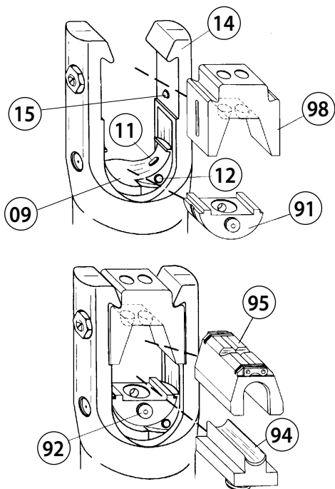
FIG. 5 DIE INSERTION - INSERTION DES MATRICES - EINSETZEN PRESSEINSÄTZE - INSERCIÓN DE LAS MATRICES - INSERIMENTO MATRICI
